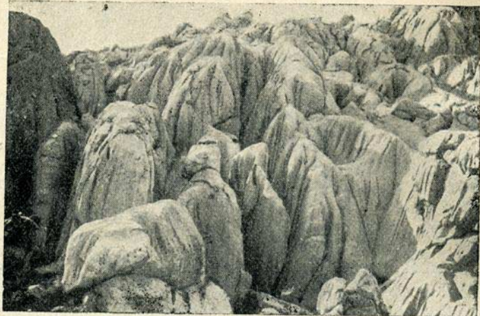
Skupina zasebno raazvijenih škrapa iznad V. Vaganca na Velebitu
