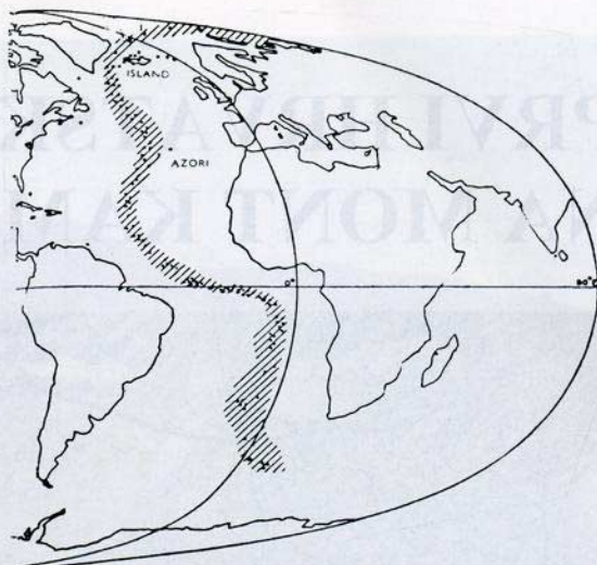
Podmorski greben uzduž Atlantskog oceana, možda ostatak nekadašnje Atlantide
