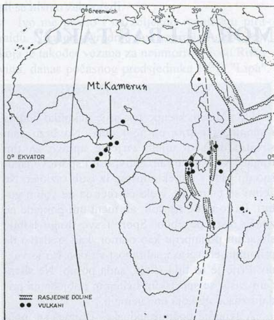
Položaj Mt. Kameruna u vulkanskom nizu ekvatorijalne zapadne Afrike
