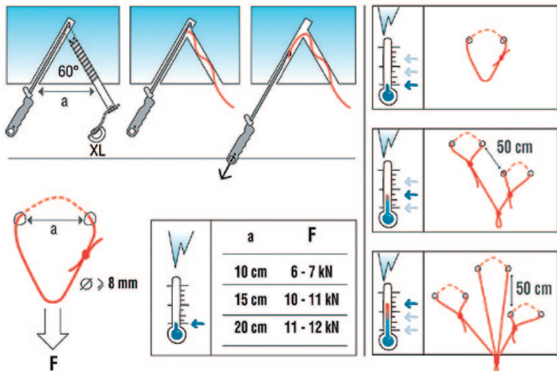
Slika 7. Izrada i nosivost horizontalnog Abalakov-sidrišta. Izvor: katalog Petzl (2008).
