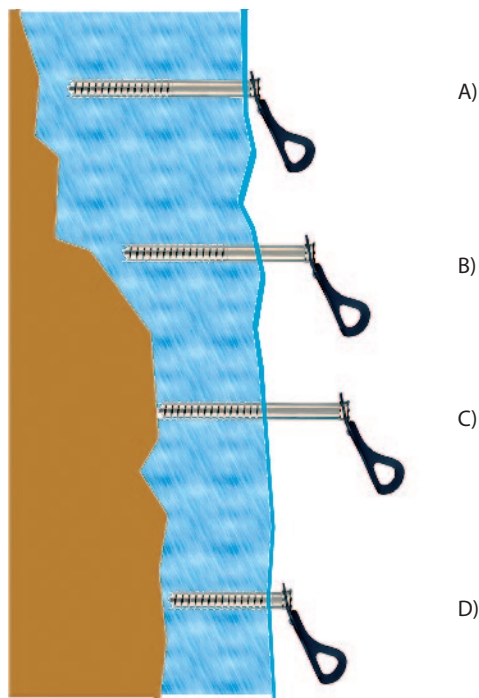
Slika 4. Debljina leda i pouzdanost lednog vijka: A) izvrsno, B) dobro ako vijak ne viri više od 5 cm, C) loše, D) vrlo dobro
