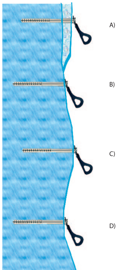
Slika 3. Postavljanje lednog vijka: A) loše: neočišćen sloj »lošeg« leda, B) dobro, C) loše: led je ispupčen, D) izvrsno: led je udubljen
