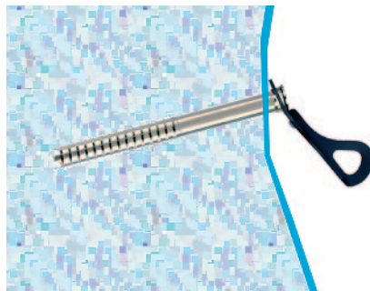
Slika 6. Kut postavljanja lednog vijka u »lošem« ledu
