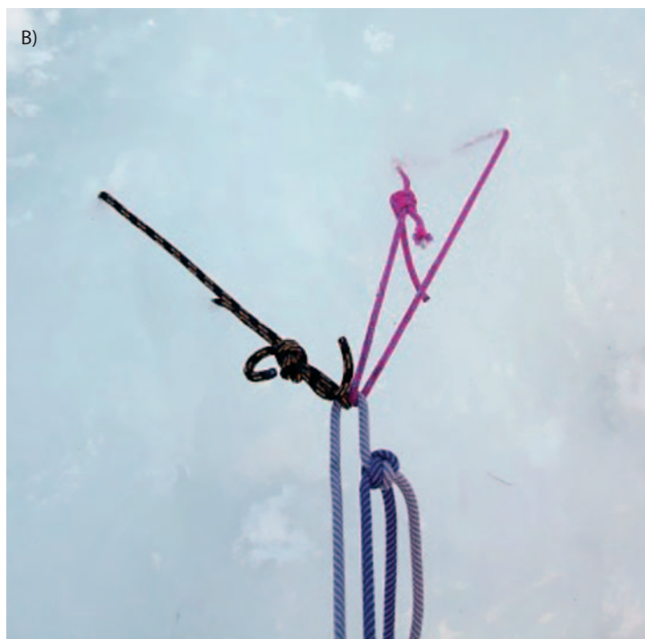
Slika 8. A) Horizontalno Abalakov-sidrište dodatno osigurano lednim vijkom, B) pronađeno horizontalno Abalakov-sidrište (desno) pojačano novim dijagonalnim (lijevo)
