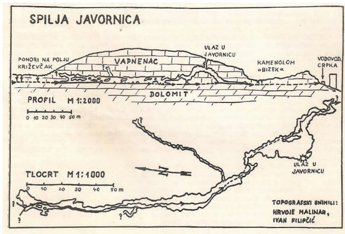
Nacrt špilje Javornice
